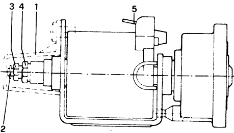
1 - Kappe 2 - Kern des Magnetantriebs 3 - Maximaldruckeinstellmutter 4 - Minimaldruckeinstellmutter 5 - Flachsteckeranschluß
